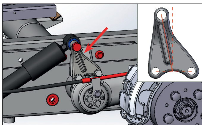
Øvre støtdemperfeste "S" (braketten er bøyd litt fremover)
