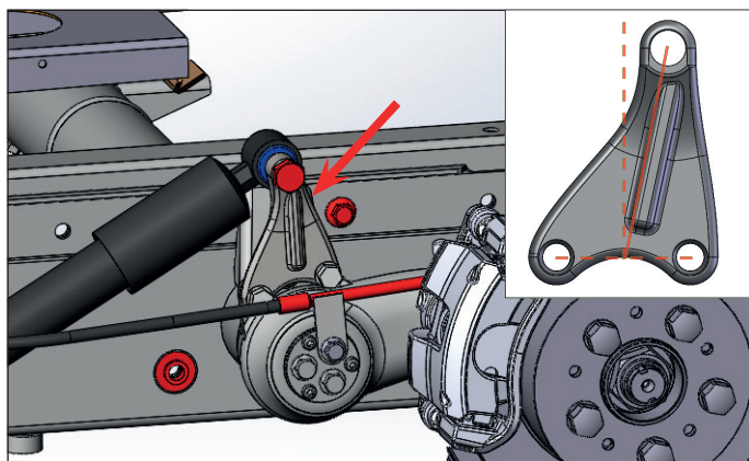
Øvre støtdemperfeste "V" (braketten er bøyd litt bakover)
