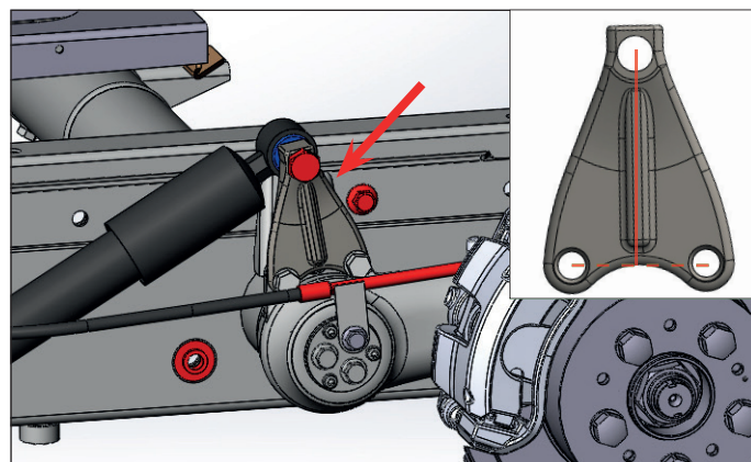
Øvre støtdemperfeste "T" (braketten er rett)
